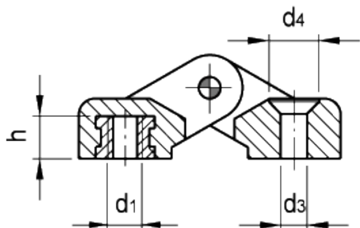
通孔 SH
