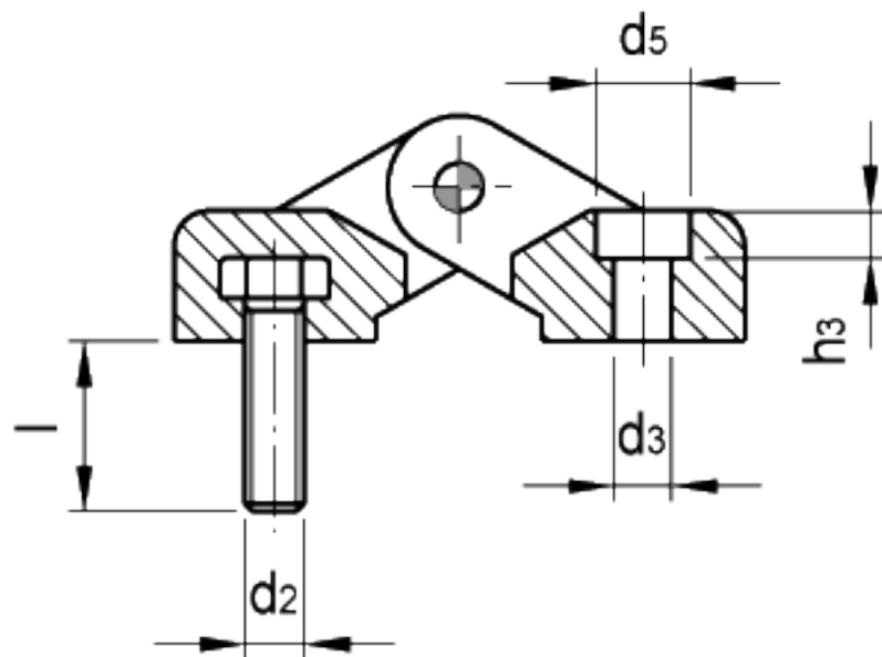
螺杆(p)/通孔CH
