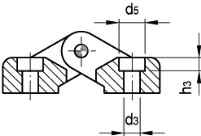
衬套 (B)
