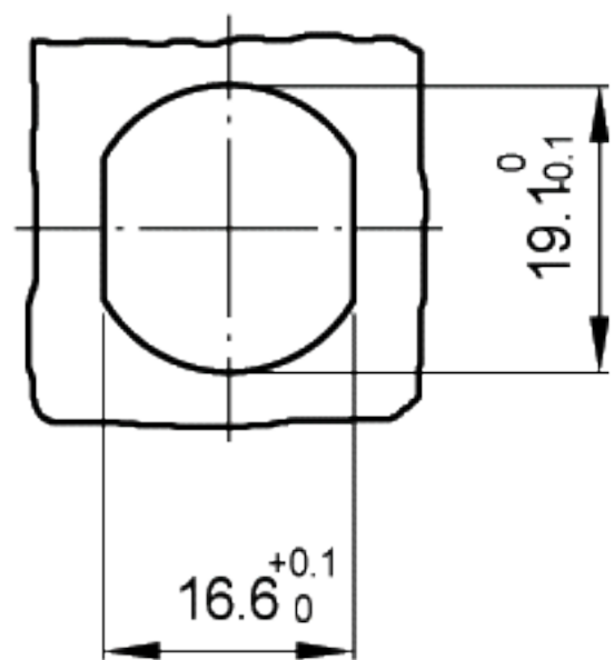
钻孔模板
