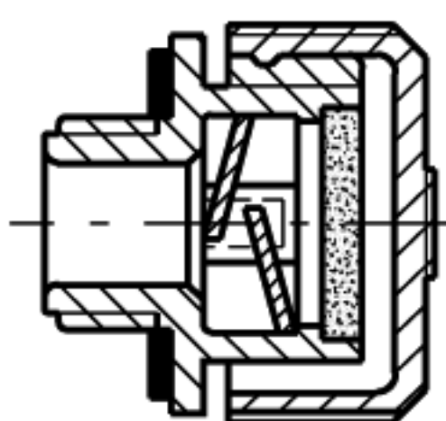
SFP+F 型 (D=31-42-57)
