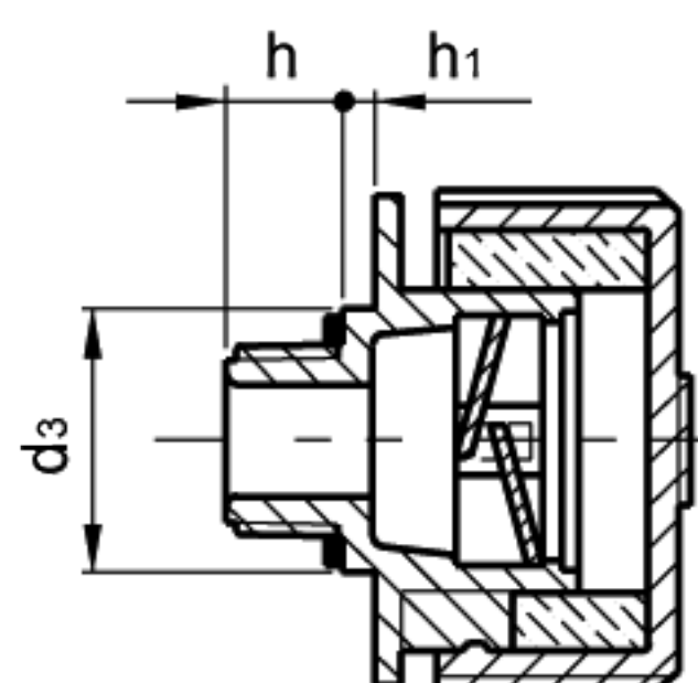
SFP+F 型 (D=70)
